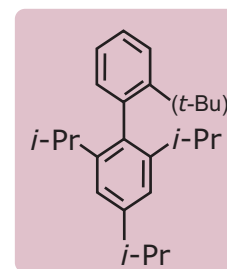
tBuXPhos
