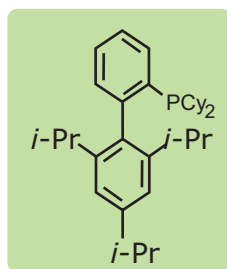
Xphos
