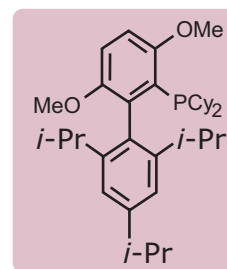
BrettPhos
