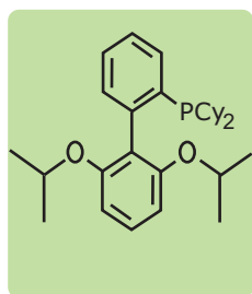
RuPhos
