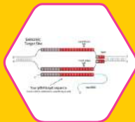
CRISPR/CAS9
